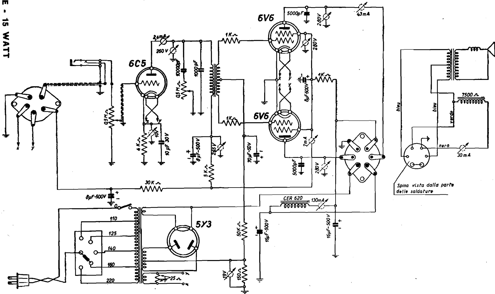
COMPAGNIA GENERALE DI ELETTRICITÀ - Amplificatore da 15 watt per centralino radio-micro-fonografico da scuola.
